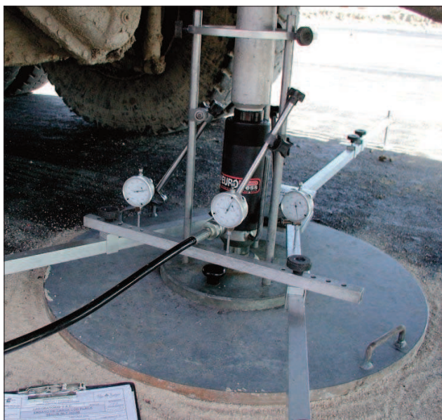
Figura 7.1 Placa de carga
