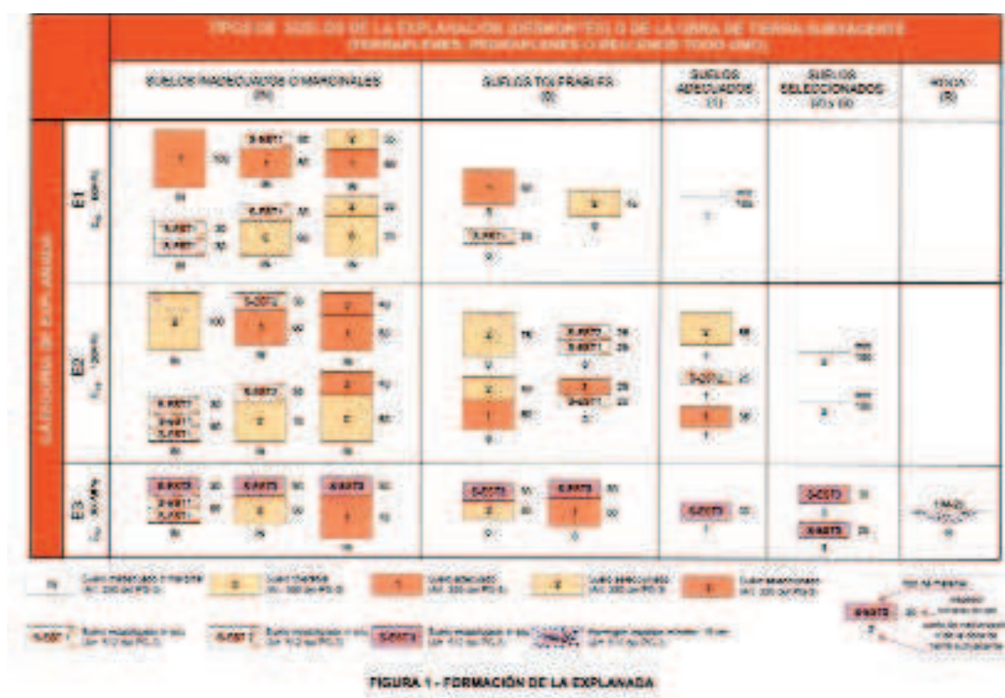
Figura 9.2 Formación de explanadas (Norma 6.1-IC)
