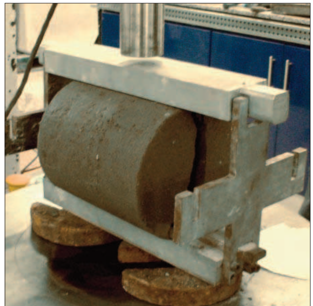
Figura 4.9 Ensayo de tracción indirecta
