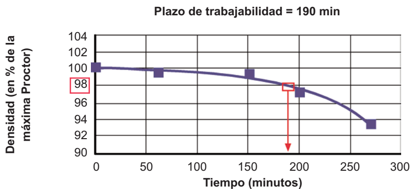
Figura 4.7 Determinación del plazo de trabajabilidad de una mezcla con cemento mediante el ensayo de compactación diferida a una temperatura de 30 °C
