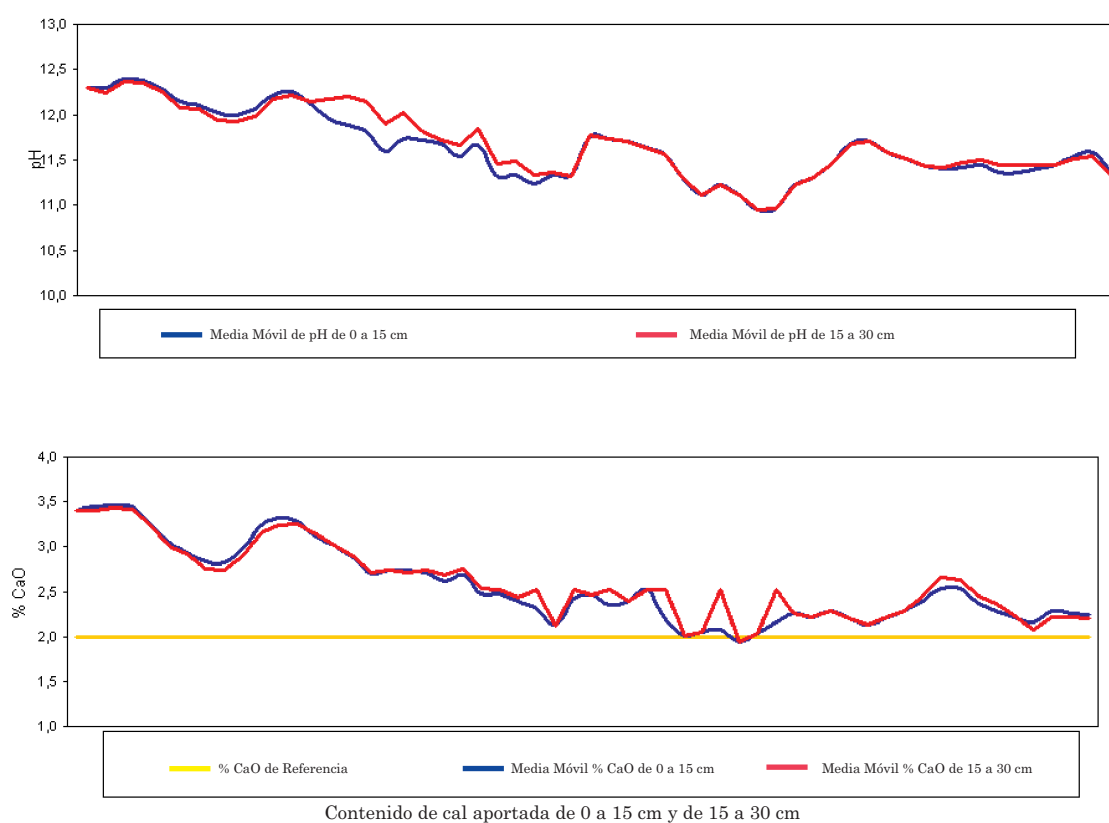
Figura 7.7 Modelos de gráficos de control
