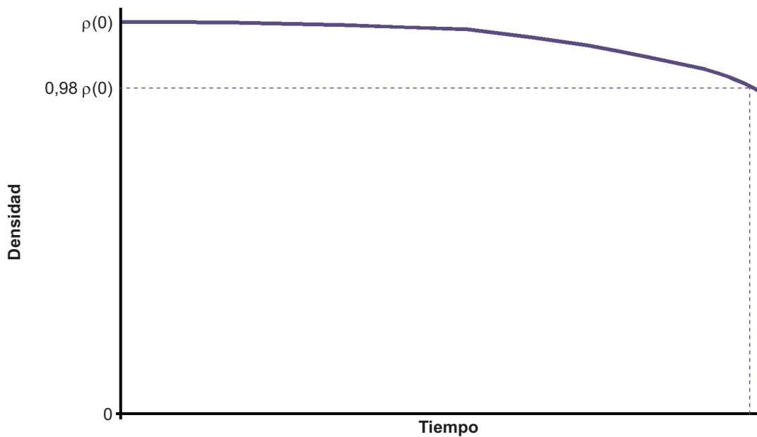
Figura 3.8 Determinación del plazo de trabajabilidad por el método de compactación diferida (norma UNE-EN 13286-45)
