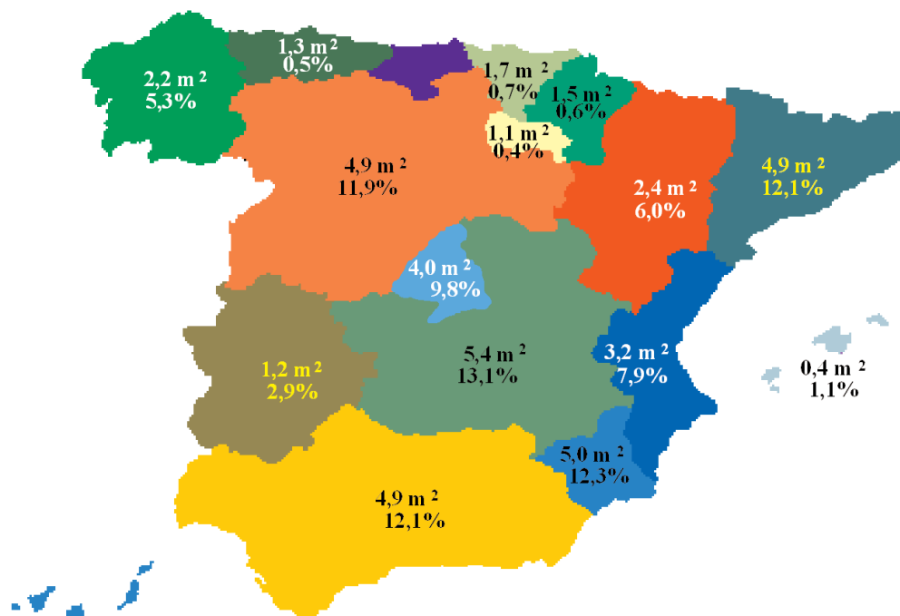
Figura 1.8 Superficie ( 10^6 \text{ m}^2 ) de explanadas estabilizadas con cemento en España en el periodo 2006 a 2007
