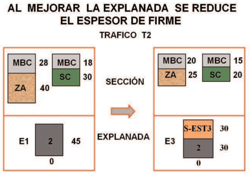
Figura 9.8 Ejemplo de diseño conjunto firme-explanada
