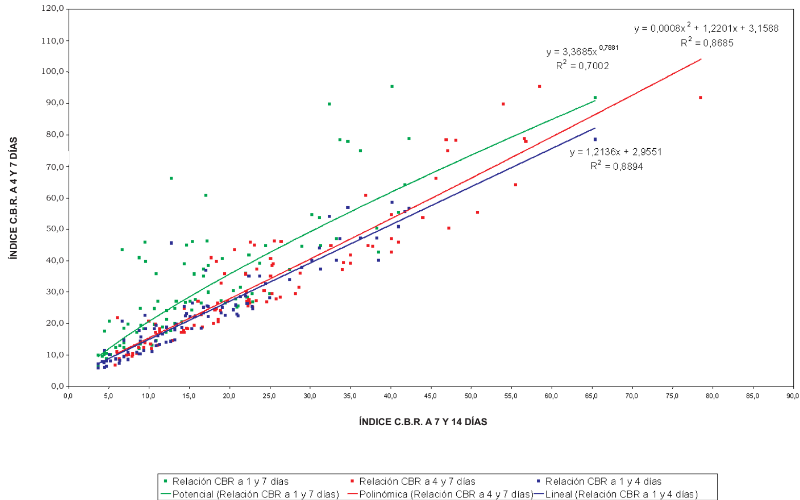
Figura 3.4 Ejemplo de evolución del índice CBR a 1, 4 y 7 días.
